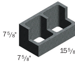
Header
