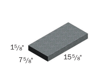
2-inch Cap
