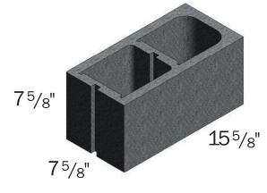
Conduit
